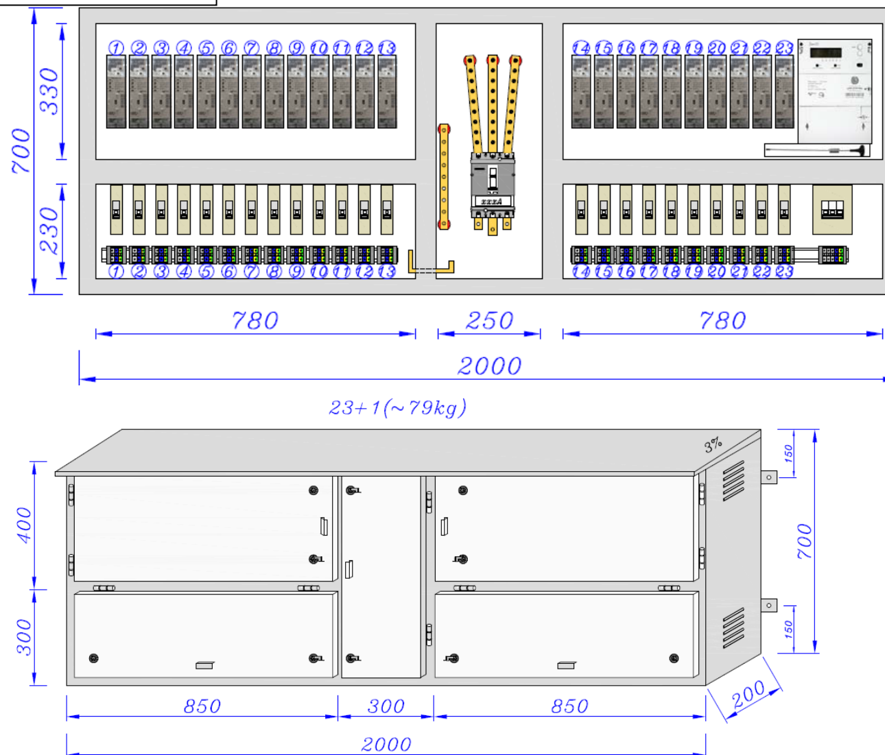
LAYOUT _ B4: 23+ 1 کتوری
